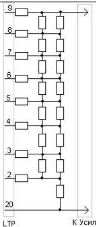
Рис.1 Схема Covox'a
